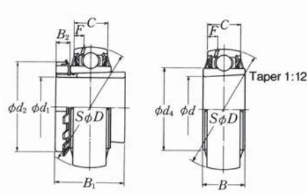
UK3...D1;H, HA, HE, HS UK3...D1
